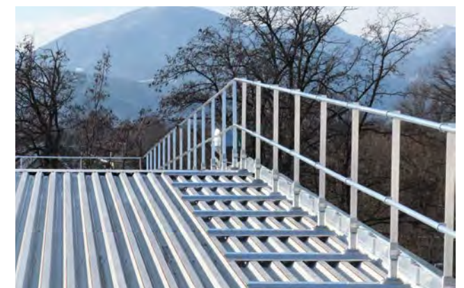
Sicherheitsgeländer Metalldach
