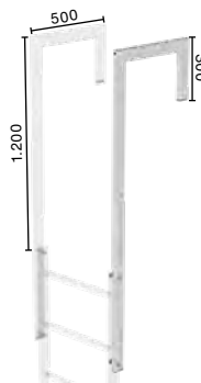
Abb. Bestell-Nr. 62049 (2 St.)
