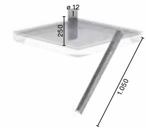
Abb. Bestell-Nr. 60954 (Flanschplatte und Strebe für Ziegelmauerwerk)
